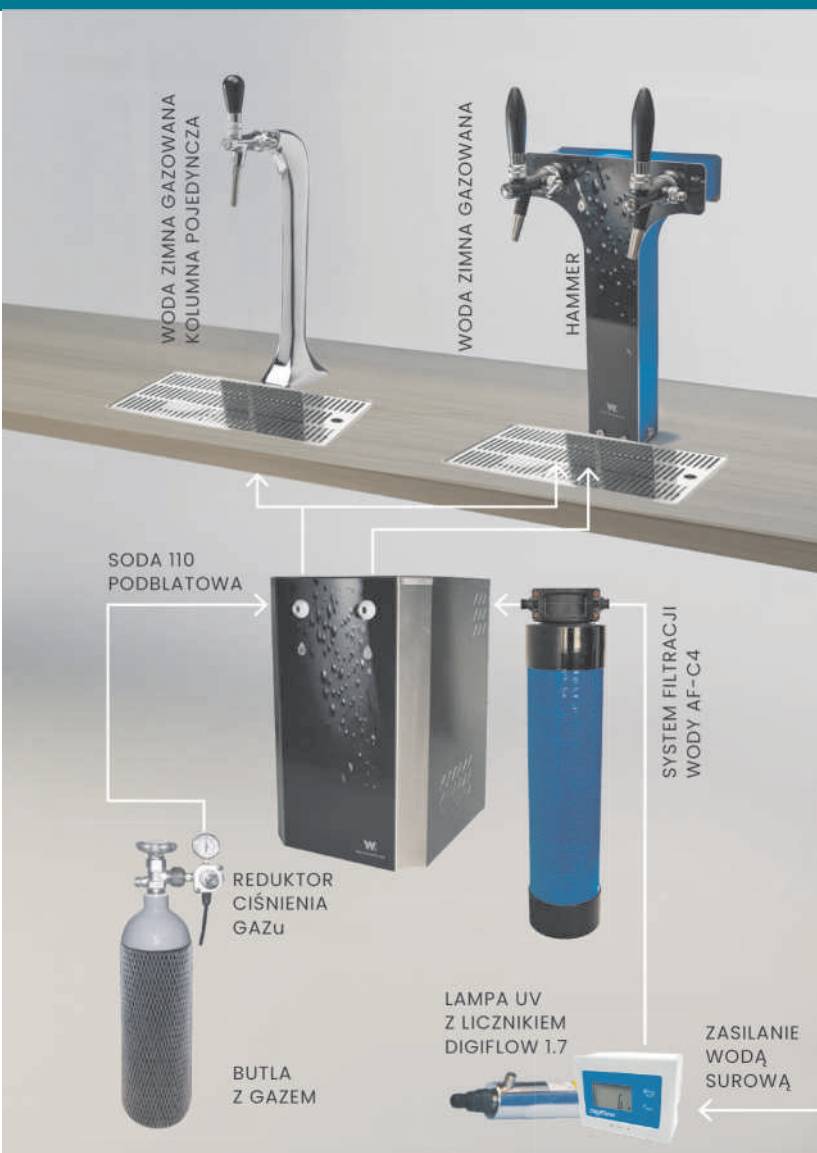
Przykładowa instalacja podpulpitowego Dystrybutora wody wraz z akcesoriami
